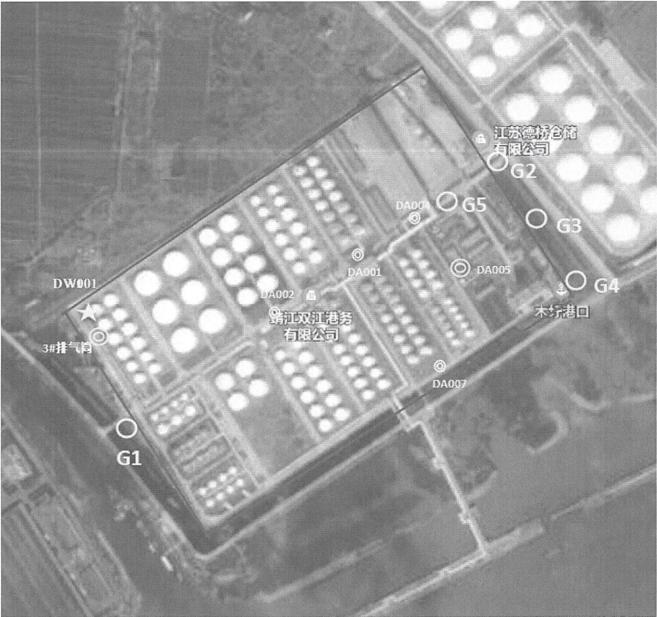
废水、废气监测点位示意简图
